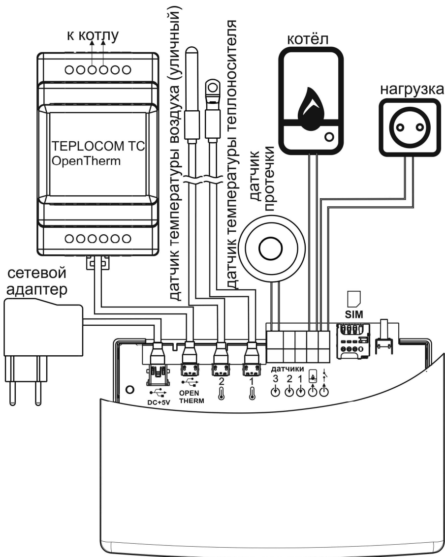
Рисунок 3 - Схема подключений
